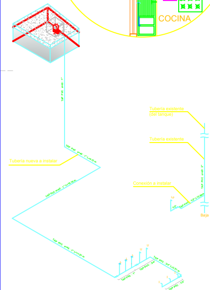
ISOMÉTRICO ESC:1:100
