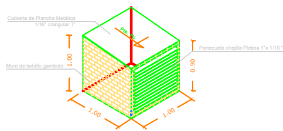
DETALLE CASETTA DE BOMBEO ESC:1:25
